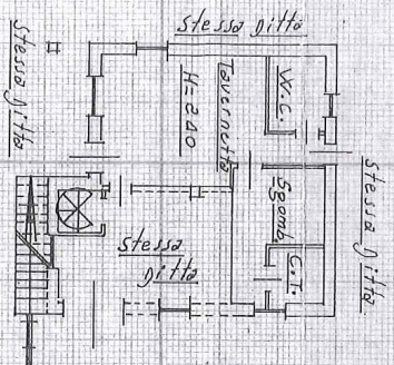
PIANTA PIANO TERRENO
