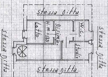
PIANTA MANSARDA
